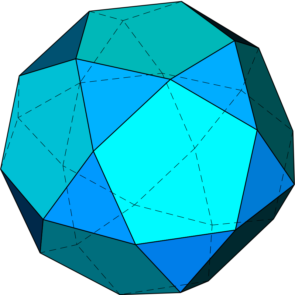
Icosidodécaèdre
