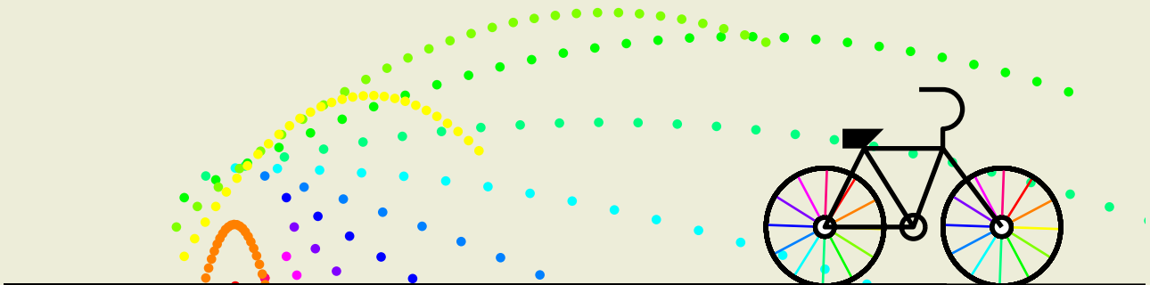
FIG. 6 – trajectoires absolues
