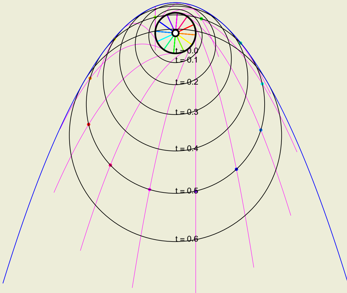
FIG. 5 – enveloppe des cercles
