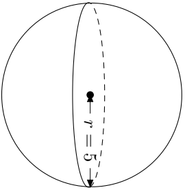
Boule
