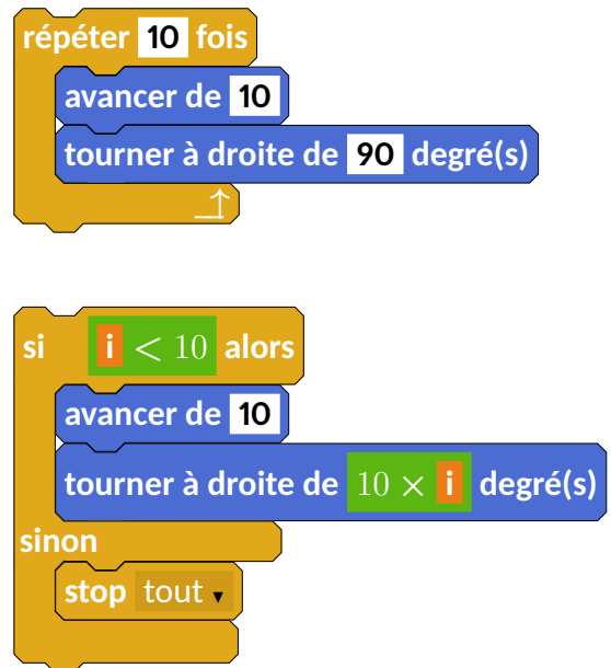
FIGURE 4 – Comparaison Scratch / METAPOST pour l’affichage des « sorties » de boucles et tests.
