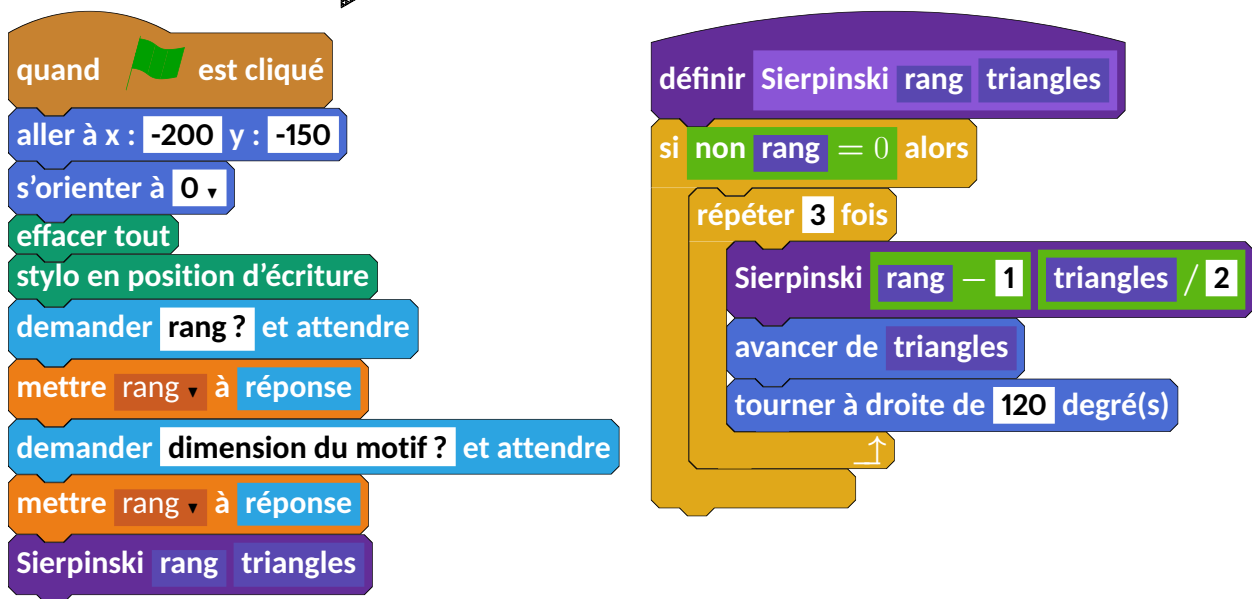
FIGURE 9 – Triangle de Sierpinski - Code Scratch et METAPOST
