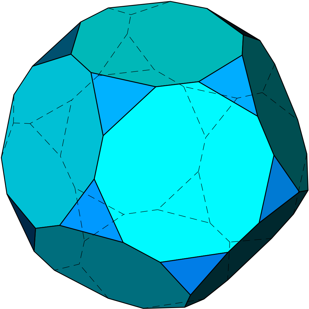
Dodécaèdre tronqué
