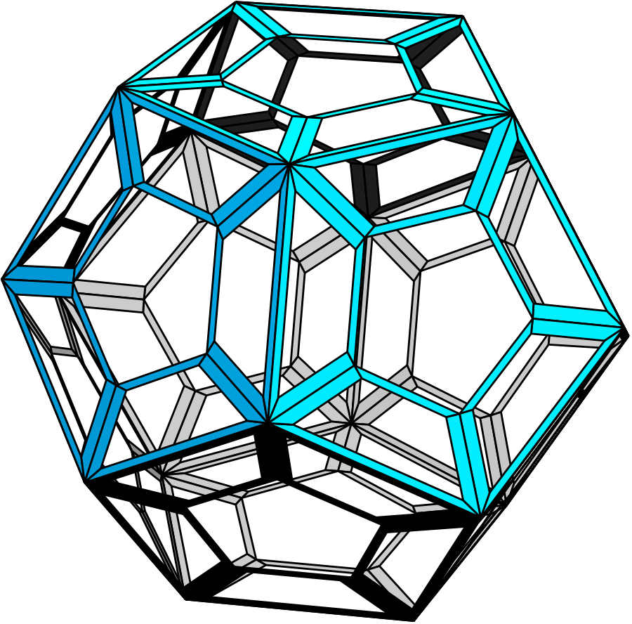
Dodécaèdre
